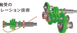
スカイピング・歯研の 3D歯面修整加工技術 (エンドリリーフ、 バイアス修整)
