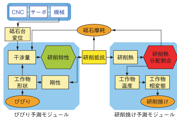
図3 加工モデル Machining model of grinding
