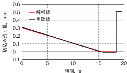
図9 切込み残り量の解析値と実験値の比較結果
