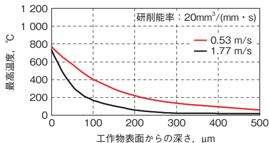
図11 工作物における最高温度の予測結果
