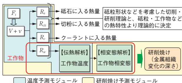
図8 研削焼けの予測手順
