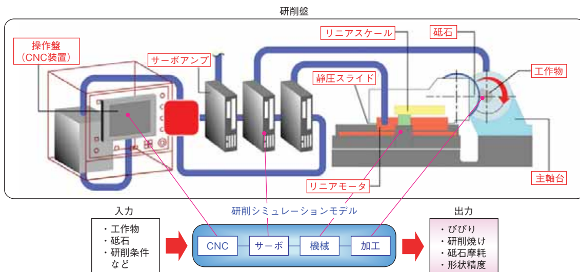
図1 研削盤トータルシミュレータの概要
