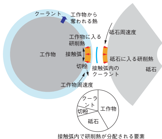
図6 研削熱の授受モデル Transfer model of grinding heat
