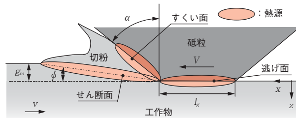
図7 砥粒研削点における単粒切削モデル Machining model with single grain at grinding point
