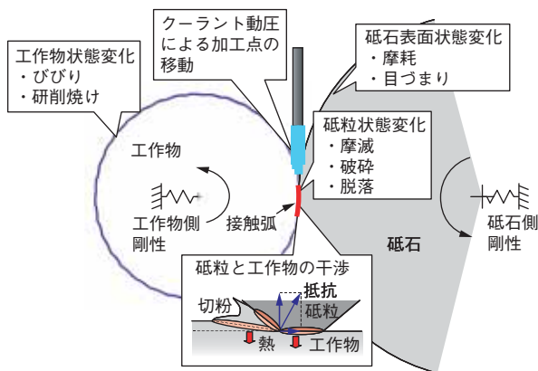
図2 研削における加工プロセス Machining process of grinding
