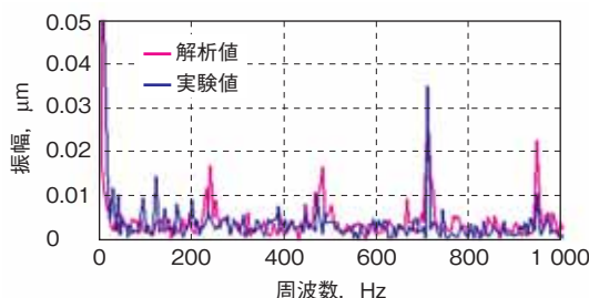
図10 工作物形状の周波数分析における解析値と実験値の比較結果
